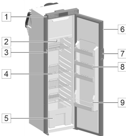
Abb. 166: 12 V-Kompressor-Kühlschrank
