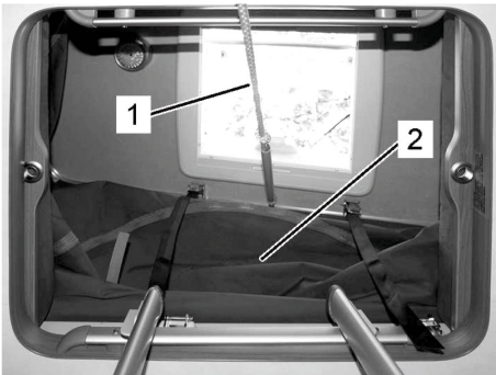
Abb. 149 Zugleine (1), Faltenbalg (2)
