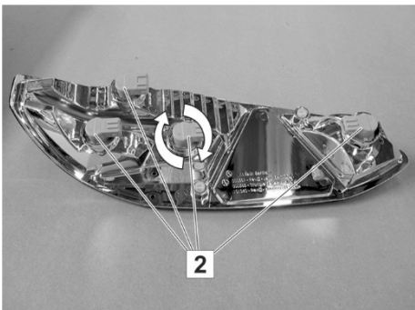
Abb. 176: Heckleuchte (Rückseite)
