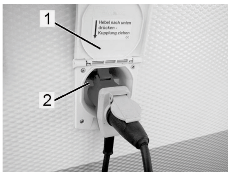
Abb. 66: Netzanschluss
