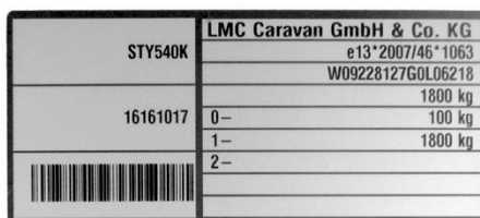
Abb. 1: Typenschild
