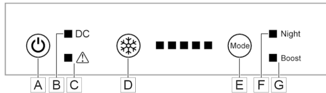
Abb. 167: Bedienelemente 12 V-Kompressor-Kühlschrank
