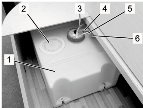
Abb. 92: Frischwassertank, Beispiel
