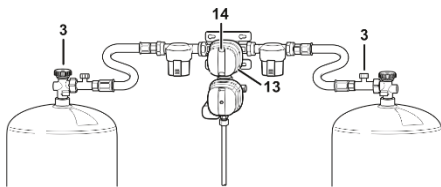
Abb. 113: Gasdruckregler-Set
