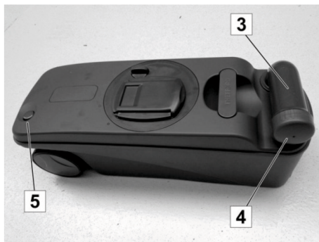
Abb. 155: Fäkaliertank entleeren
