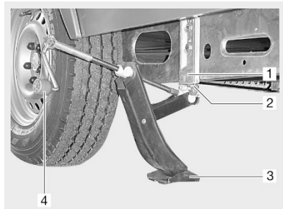
Abb. 172: Wagenheber AL-KO
