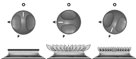
Abb. 161: Stellungen der Bedienelemente: AUS, Hochflamme, Sparflamme
