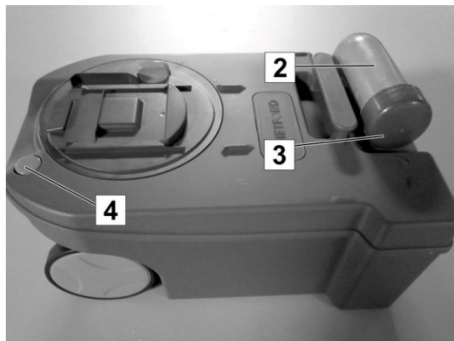
Abb. 158: Fäkalientank entleeren
