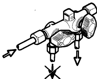
Abb. 86: Absperr- und Freigabestellung
