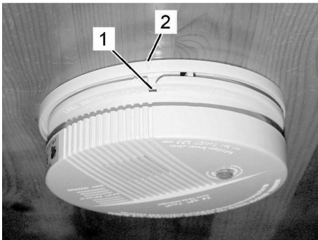
Abb. 116: Gehäuse ansetzen
