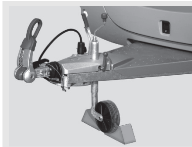
Abb. 218: Stützrad sichern
