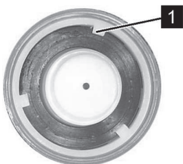
Abb. 107: Drehverschlussdeckel, innenseitig
