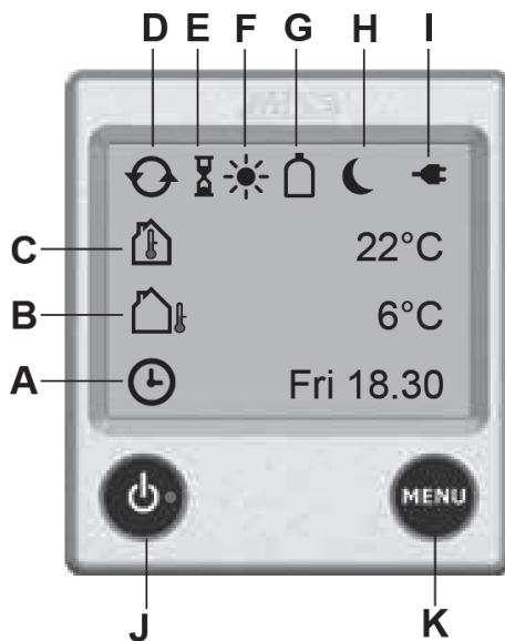
Abb. 162: Bedienelemente
