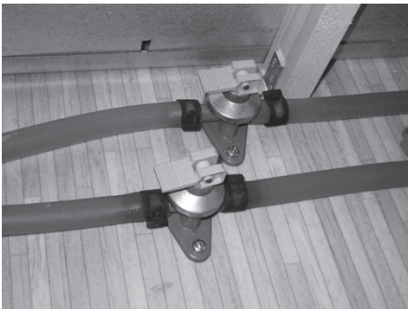
Abb. 178: Ablassventile geschlossen
