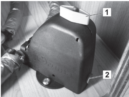
Abb. 111: Sicherheits-Ablassventil offen
