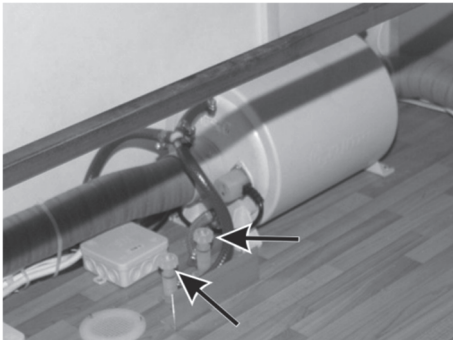
Abb. 101: TRUMA-Therme und Wasserablassventile
