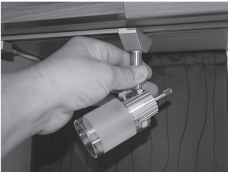
Abb. 191: LED-Strahler versetzen
