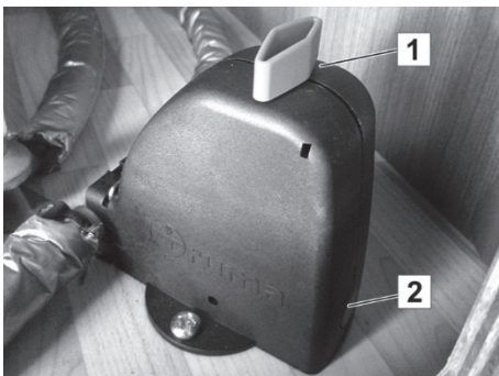
Abb. 112: Sicherheits-Ablassventil geschlossen
