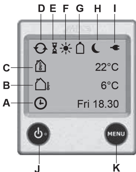
Abb. 88: Bedienelemente
