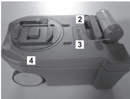
Abb. 203: Fäkalientank entleeren
