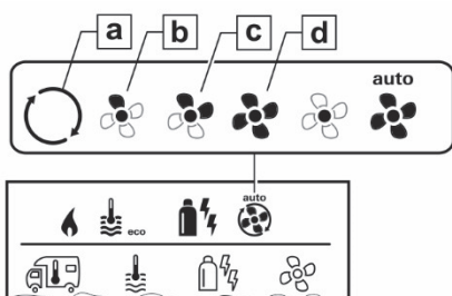
Abb. 147: Symbol Gebläsestufe
