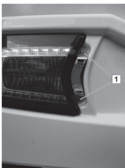
Abb. 226: Heckleuchte anbringen
