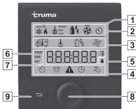
Abb. 140: Digitale TRUMA-Bedieneinheit CP Plus
