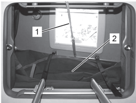
Abb. 194 Zugleine (1), Faltenbalg (2)
