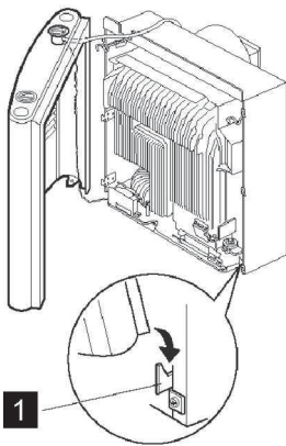
Abb. 134: Heizverkleidung aufgeschwenkt
