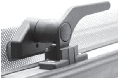
Abb. 26: Belüftungsstellung
