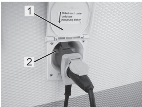
Abb. 105: Netzanschluss
