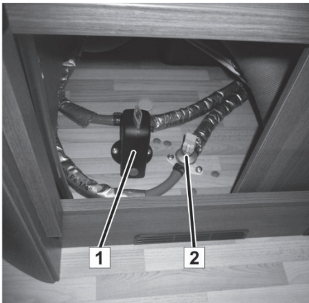
Abb. 110: Ablasventile TRUMA-Combi-Heizung
