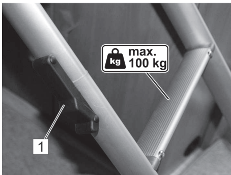
Abb. 193: Verriegelung (1) der Aufstiegsleiter
