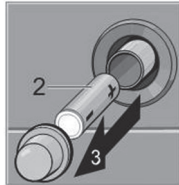
Abb. 216: Batteriewechsel bei Batterie-zünder (nur wenn vorhanden)
